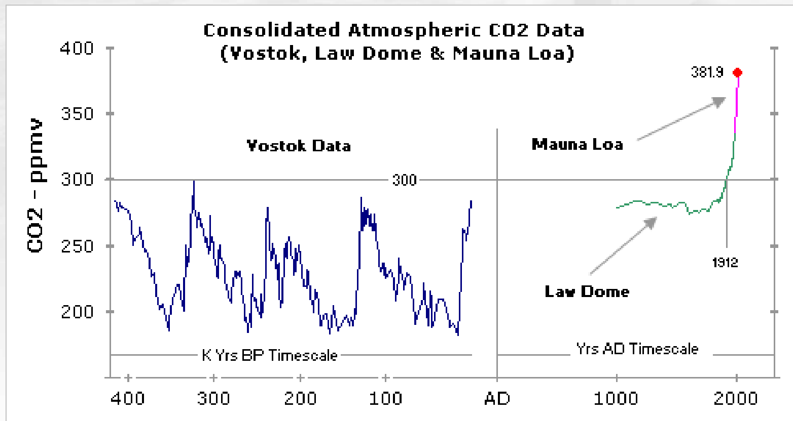
Concentration de CO2 dans l'atmosphère -400 000 ans à aujourd'hui
