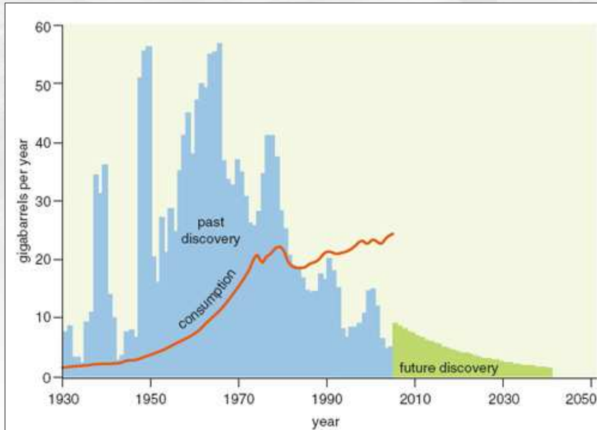
Découvertes et consommation de pétrole depuis 1930
